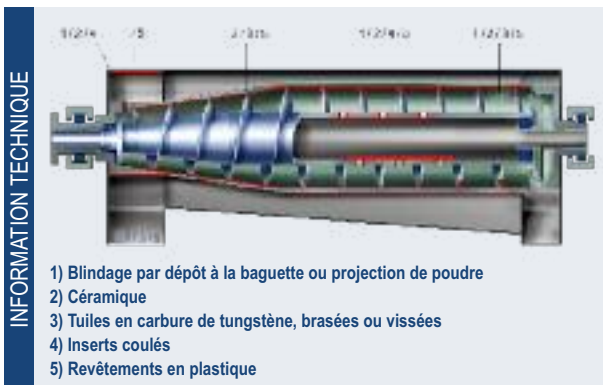
Éléments remplaçables de protection contre l'abrasion
