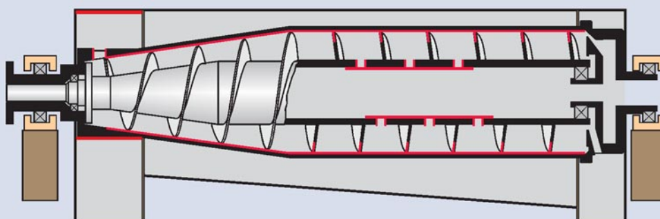
Secciones marcadas en rojo – dispositivos de protección antidesgaste reemplazables
