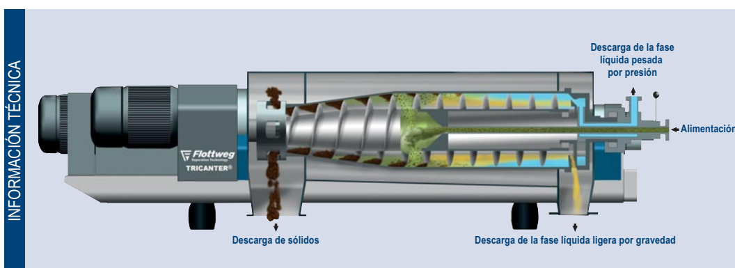
TRICANTER® FLOTTWEG (DECANTER DE TRES FASES)
