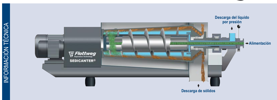
SEDICANTER® FLOTTWEG
