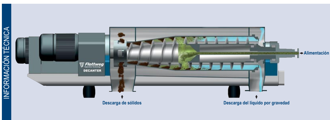
DECANTERS FLOTTWEG para la separación de sólidos de mezclas líquidas con descarga por gravedad de la fase líquida (concentrado)
