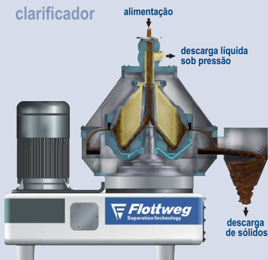
Clarificador Flottweg para separação de sólidos de líquidos
