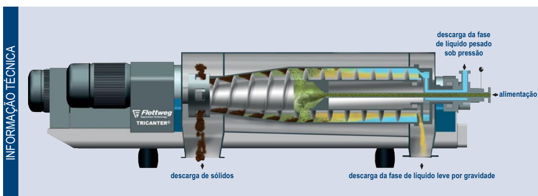
Tricanter® Flottweg (decanter de três fases)
