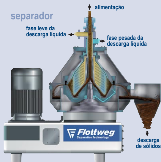
Separador Flottweg para a separação de dois líquidos imiscíveis com separação simultânea de sólidos
