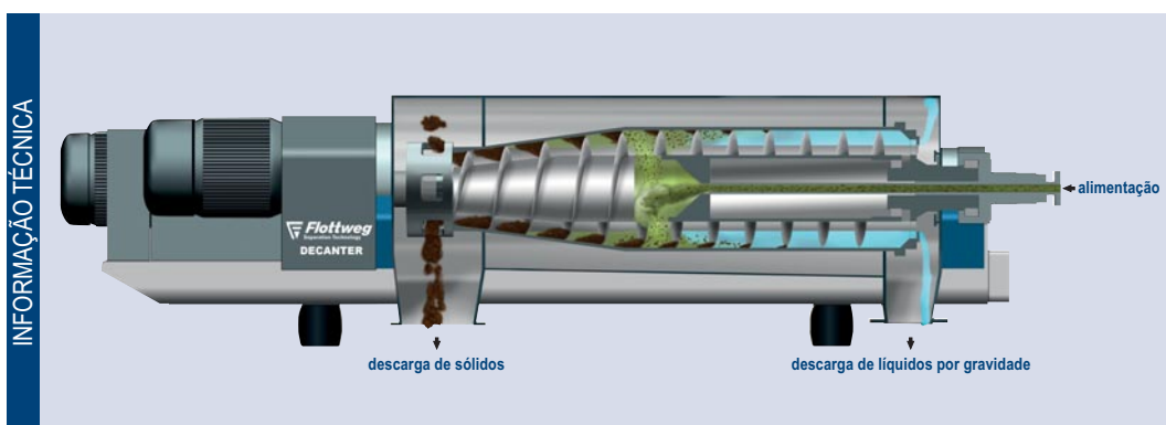
Decanter Flottweg para a separação de sólidos de líquidos com descarga por gravidade da fase líquida (concentrado)
