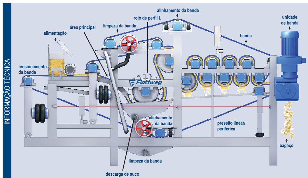
Como a prensa de banda funciona
